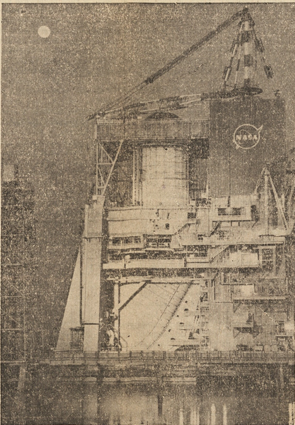
SATURNA PRESKUŠAJO — Saturn V je doslej največja in najmočnejša ameriška raketa. Pognal bo na pot proti Luni vesoljsko vozilo Apollo, kadar bo za to vse pripravljeno. Sedaj preskušajo tako raketo kot vesoljsko vozilo. Prvi poskusni polet bo enkrat v prihodnjem letu. Na sliki vidimo naprave za preskušanje rakete v NASA središču v Mississippiju.
