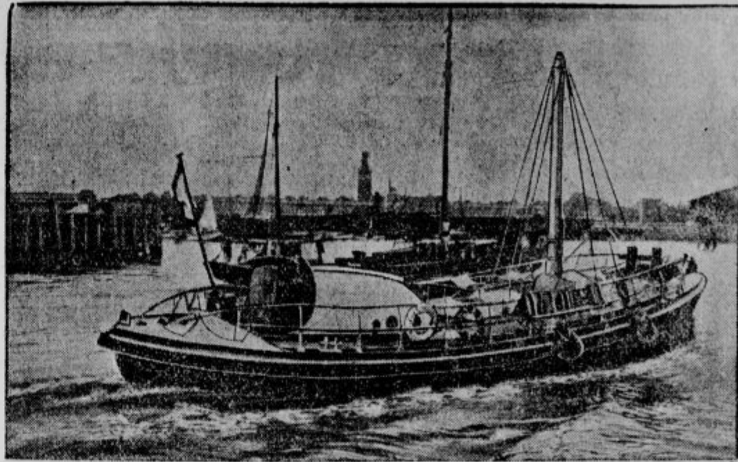
Cuxhaven ima najmodernejši rešilni čoln v Nemčiji. Sedemnajst metrov dolg rešilni čoln »Richard C. Crogmann« je pravkar nastopil svojo službo na rešilni postaji v Cuxhavnu. Čoln ima dva motorja z močjo 250 R. S. in doseže hitrost 11 morskih milj. V njem je prostora za 70 oseb.
