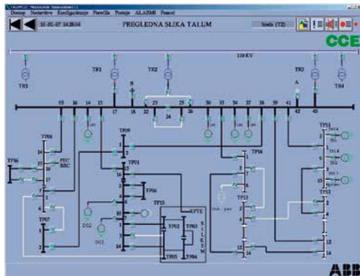
Enopolna shema 10 kV distribucijskega omrežja ZDS Talum
