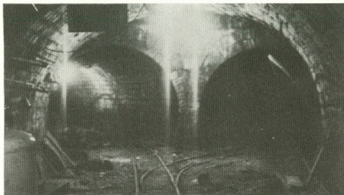
Novo križišče v okviru izgradnje NOP na koti -47 v vzhodnem, še ne do kraja izdelanem prekopu prekopne zveze z izvažalnim jaškom Nove Preloge (imenujejo ga tudi žep) je zgrajeno in je v njem treba le še dokončati montažo opreme.
