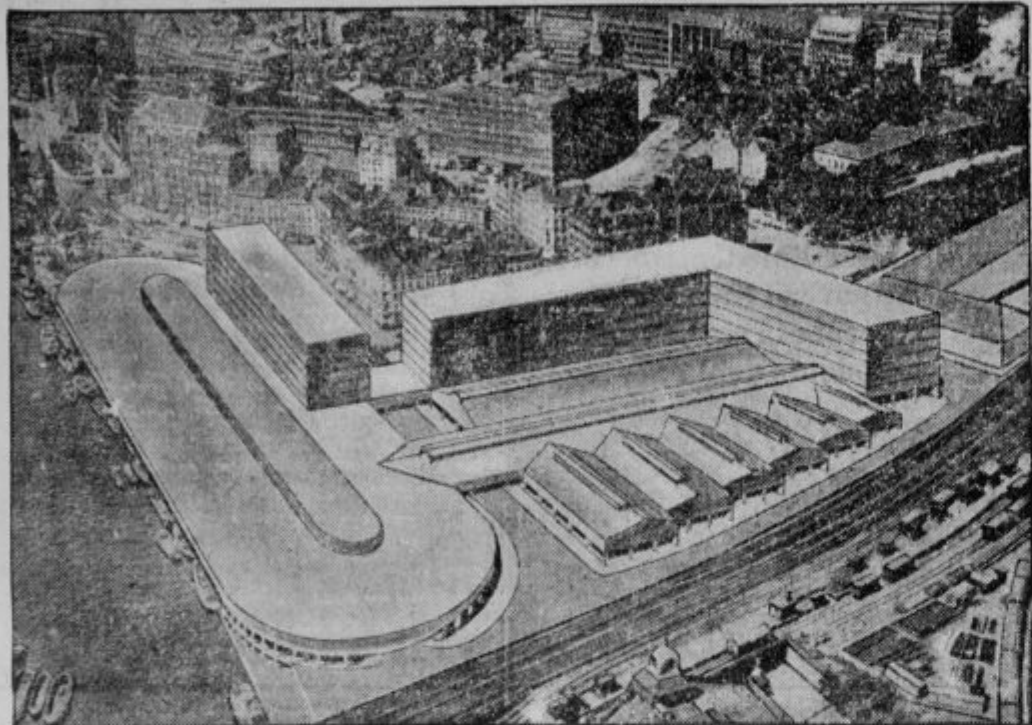
Največjo tržnico Evrope grade v Hamburgu. Tržnica bo malo mesto zase. Zgrajena bo tako, da bodo lahko ladje blago izlagale direktno v tržnico.
