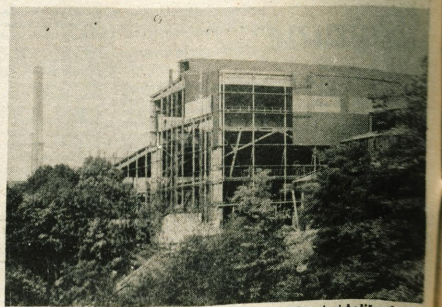
JESENICE — Ena največjih investicij za razširitev in izboljšanje materialne osnove v jeseniški železarni je prav gotovo izgradnja novega obrata kontiliva. V njem bodo namreč iz tekočega jekla, pridobljenega v jeklarni, vlivali gredice za vložek v žični valjarni. — B. B.
