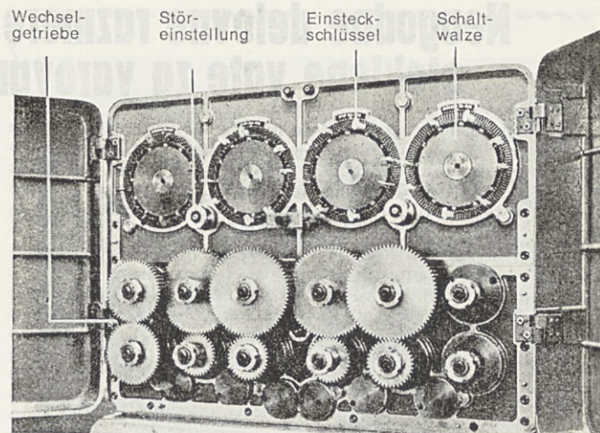
Programator na stroju za efektne sukance
