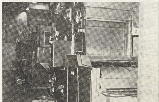
V bombažni čistilnici so remontni delavci prestavili otepalnik Platt in ga namestili pred baterjem v prizidku čistilnice.
