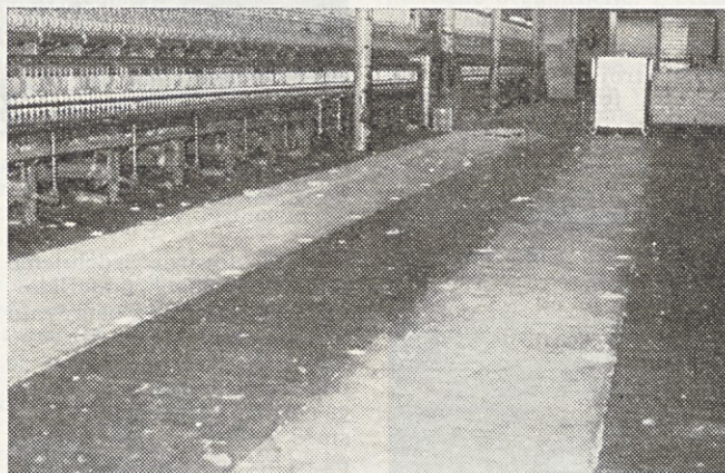
V predilnici bombaža smo demontirali 2 prstančna predilna stroja. Na to mesto bomo postavili brezvretenska predilna stroja BD-200.
