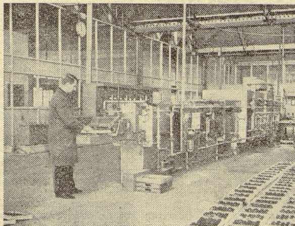
Iz obrata »Feritex« v Stegnah — delavec pri sintranju jader za odklonske tuljave v televizorjih
