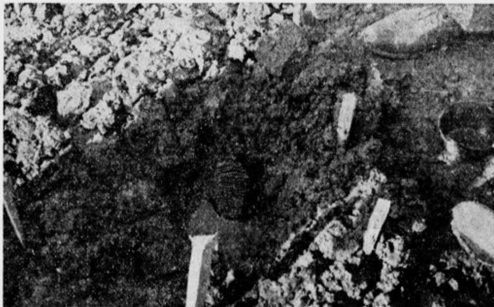
V glini ležeči mamutov kočnik. Valovite zareze dobro označujejo ploskev zoba, s katero je mlec mamut brano.
