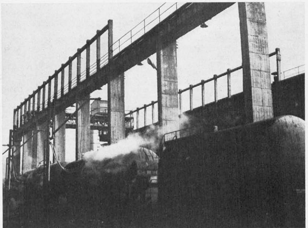
Črna energija
