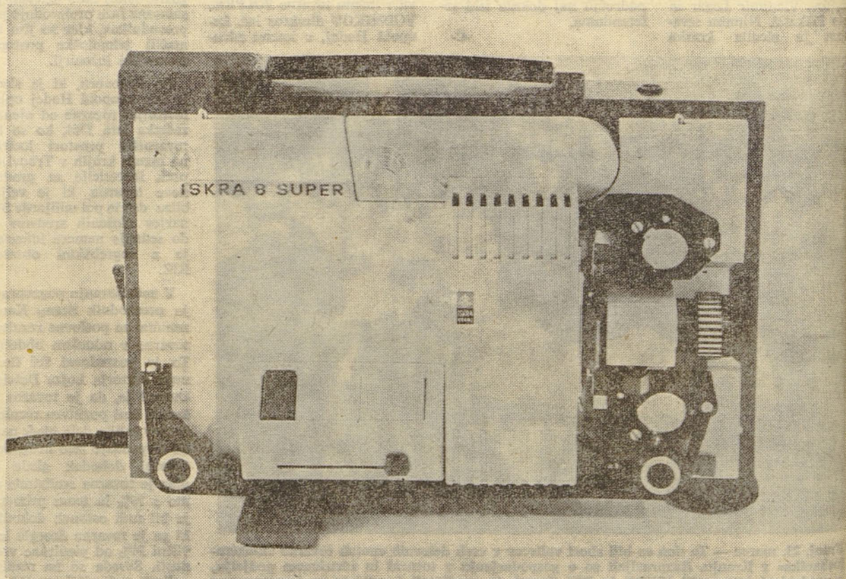
Takšen je zunanji izgled našega novega 8-milimetrskega Super kinoprojektorja. Glede na svojo lično obliko si je pridobil mednarodno priznanje, kar mu bo tudi odprlo pot v izvoz. Ta projektor je eden izmed pomembnih rezultatov ISKRE
