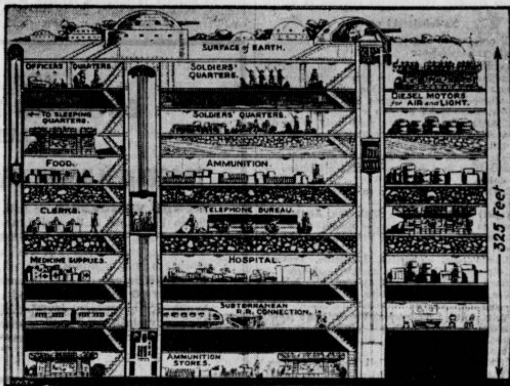
Prerez skozi Maginotovo črto
