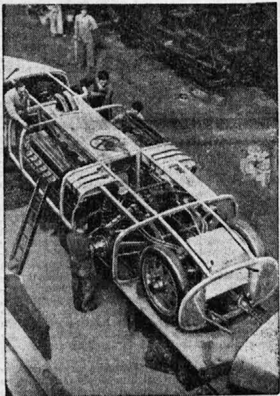
Najnovejši dirkalni avtomobil, ki so ga pred nedavnim zgradili Angleži in s katerim bodo poskušali prekositi dosedanj rekord v hitrostni vožnji. — Motor tega avtomobila ima 3000 konjskih sil
