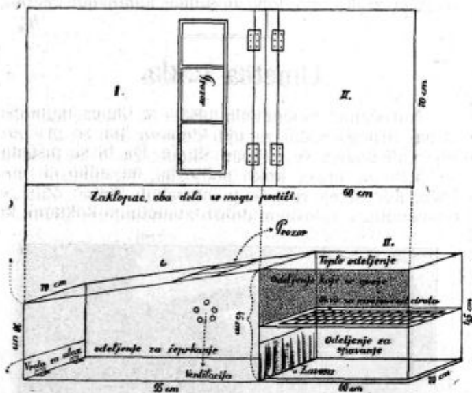
Slika 22. Umetna kokla. Načrt s pogledom odzgoraj in od strani.
