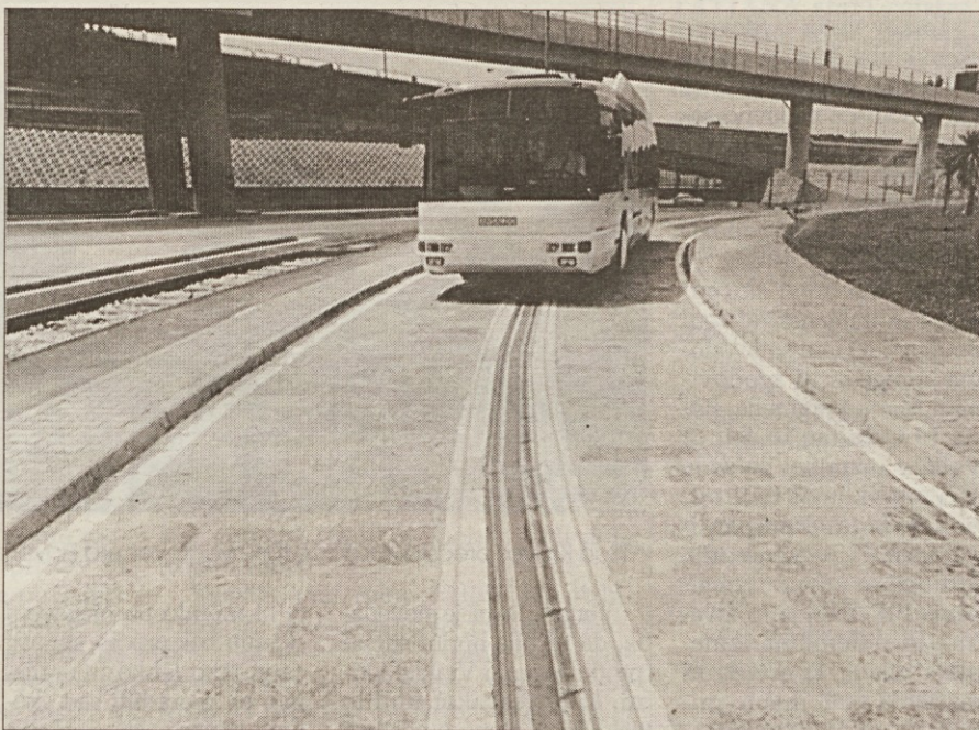
Pod avtobusom vrste stream teče plošča, prek katere vozilo črpa električni tok.
