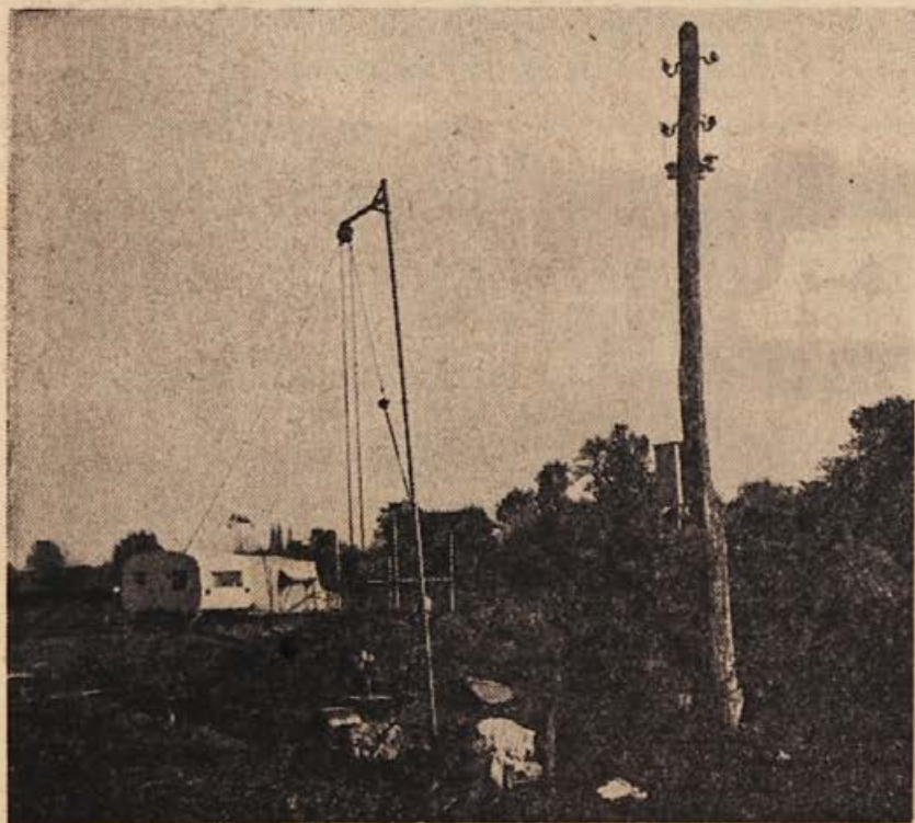
Električna lopata oz. plug, izdelek SGP »Tehnika« v Ljubljani
