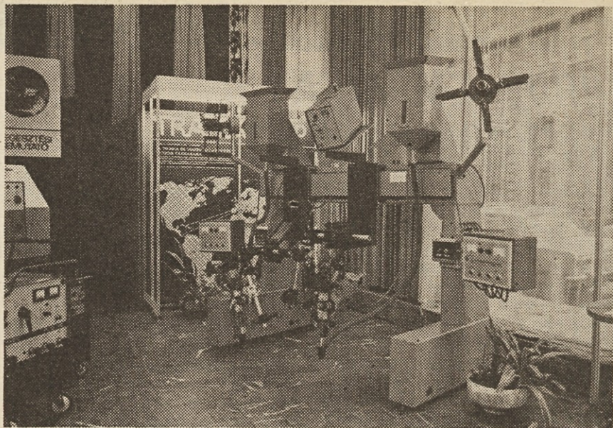
Portalni avtomat za varjenje profilov s štirimi gorilniki (slika 3).
