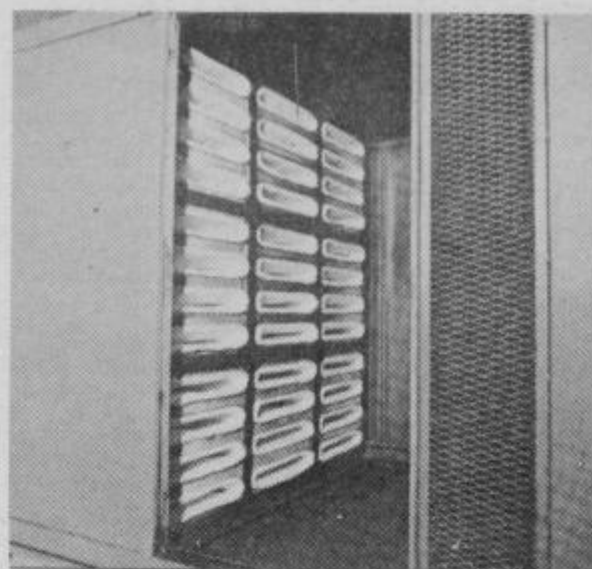
KOFIL FF 15/500 za fino filtracijo v obliki vreče
