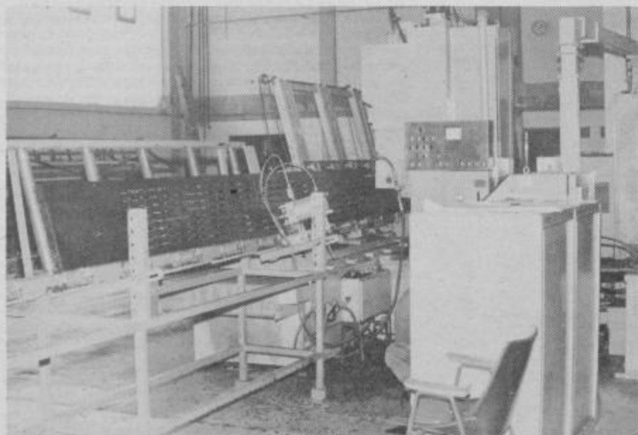
Proizvodnja sesalnih plastičnih oblog za papirno industrijo na avtomatiziranem in računalniško programiranem stroju v TOZD KOTERM.
