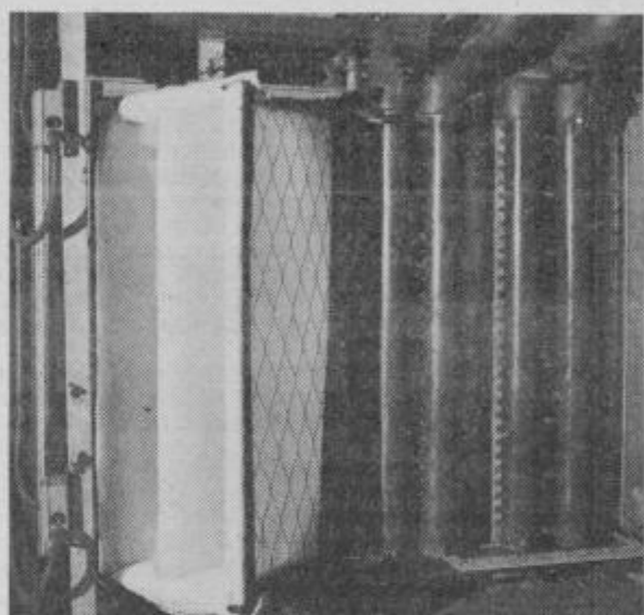
KOFIL F 10 300 kot predfilter v farmacevtski industriji
