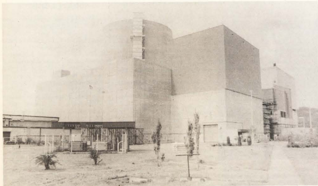
NUKLEARNA ELEKTRARNA KRŠKO je prva jedrska elektrarna v Jugoslaviji. Njene moč na pragu je 632 MW (Zwentendorf naj bi imel 700 MW). Opremljena je z Westinghousovim lahkovodnim tlačnim reaktorjem toplotne moči 1882 MW. Elektrarna je priključena na 380 KV omrežje za napajanje potrošniških središč v Socialistični republiki Sloveniji in Hrvaški. Proizvodnja električne energije v Krškem znaša letno približno 4 TWh, kar je okoli 20% električne energije proizvedene v Sloveniji in Hrvaški.
