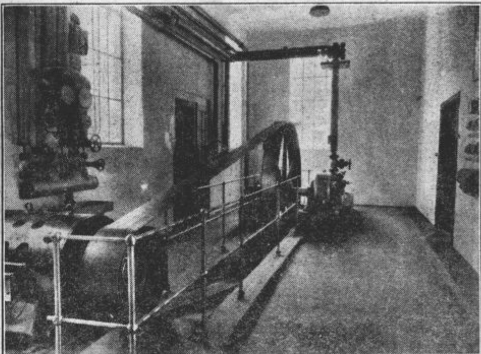
Kompresor najnov. tipa v strojnici poleg hladilnice
