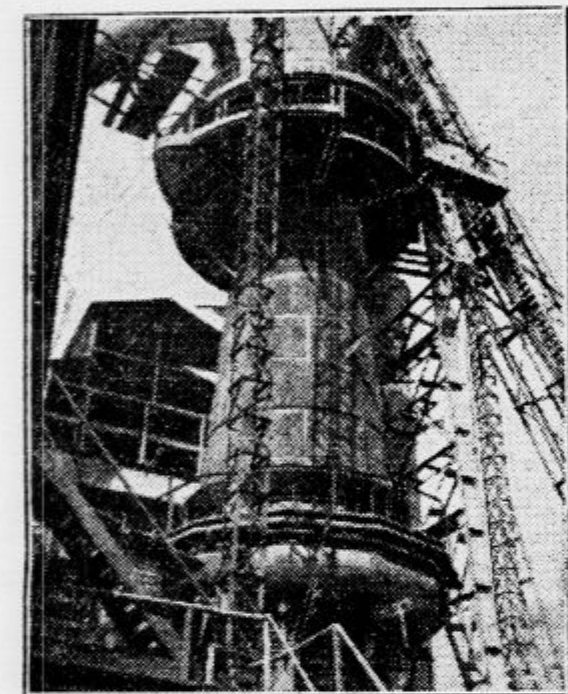
Drugi moderni plavž v železarni KID na Jesenicah
