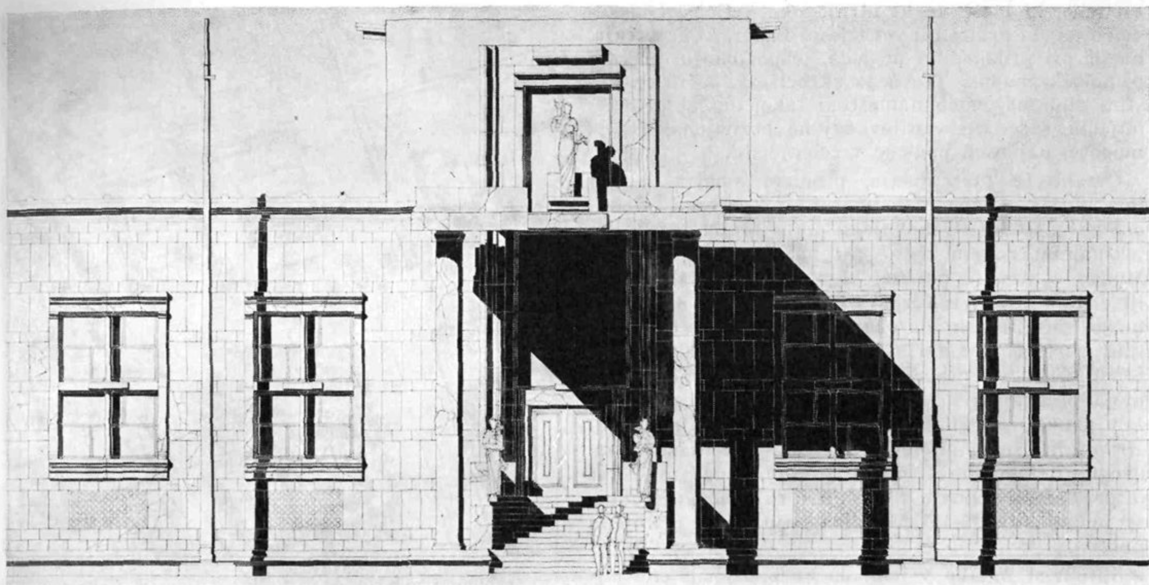
NAČRT SREDNJEGA DELA GLAVNEGA PROČELJA MODERNE GALERIJE
