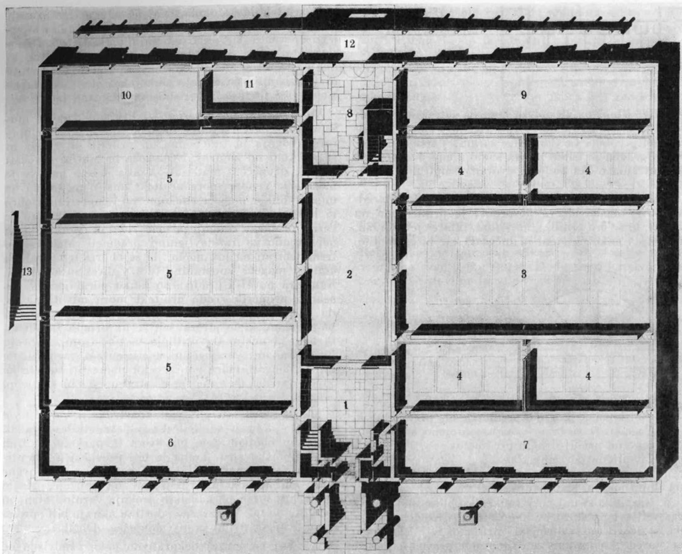
AKSONOMETRIČNI POGLED NA TLORIS MODERNE GALERIJE
