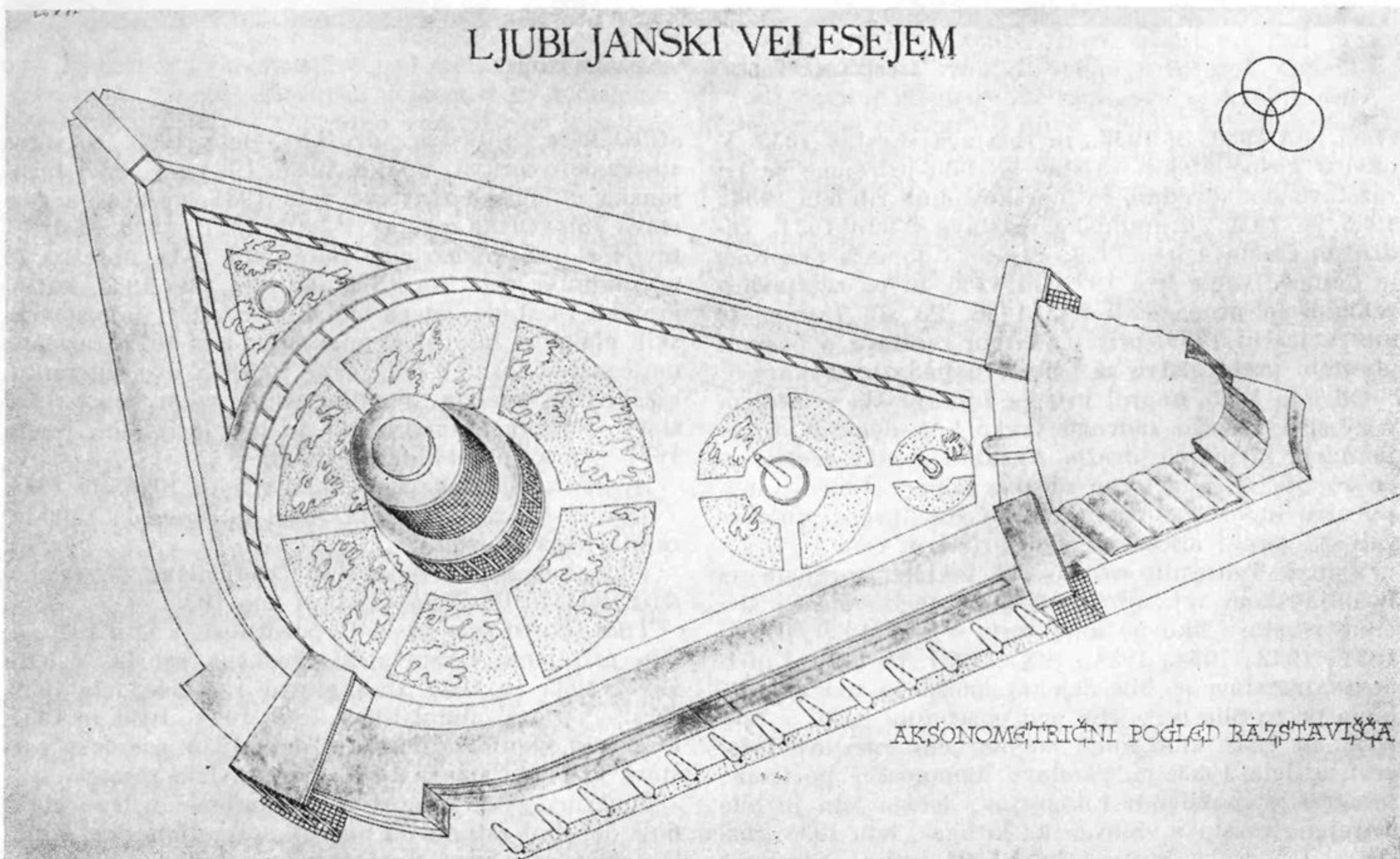
ARH. GLANZ, AKSONOMETRIČNI POGLED NA PROJEKTIRANI LJUBLJANSKI VELESEJEM
