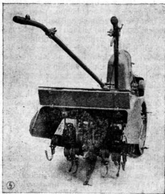
Slika 17. Freza ali stroj za drobljenje zemlje. Na stroju je videti predvsem pripravo za rezanje in drobljenje zemlje z dotičnim pokrovom. Za ročicama se vidi motor, na desno od njega pa vozno kolo.
