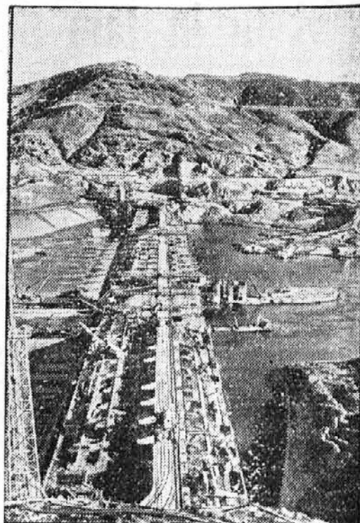
Dela pri graditvi velikega nasipa, ki bo uravnaval tok reke Kolumbije v Ameriki, hitro napredujejo. Dozdaj so porabili že okrog 4 milij. kubčnih metrov cementa, približno toliko pa ga bodo morali še, preden bo nasip, ki bo visok 60 metrov, dograjen
