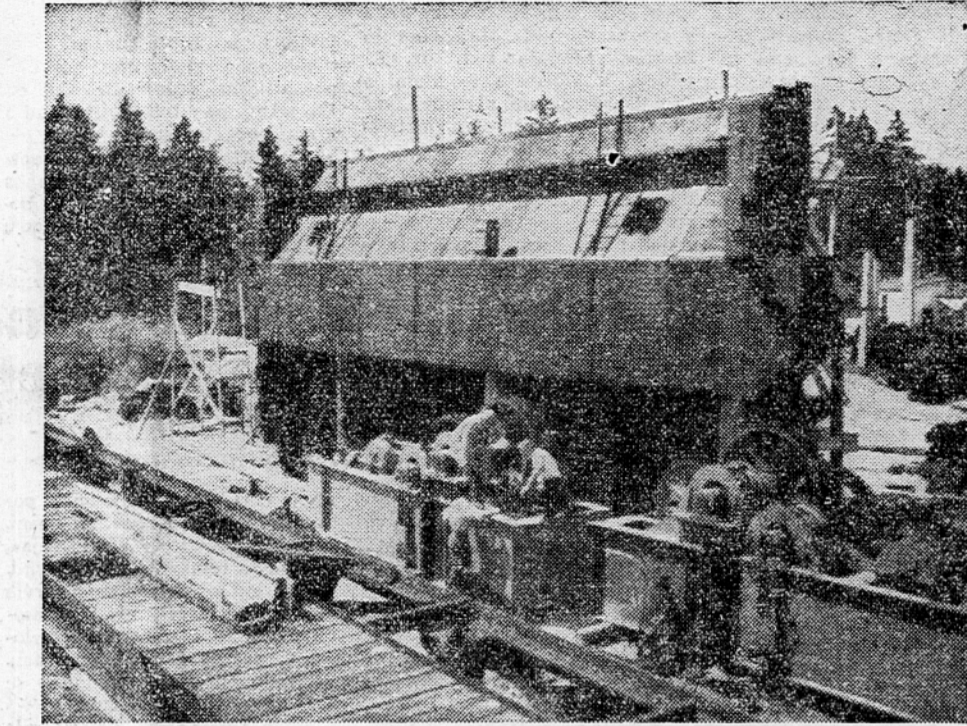
Monteži in delavci marberske »Hidromontaže« so za hidroelektrarno v Medvodah sestavili ogromno, nad 100 ton težko kovinsko zapornico. Z žerjavom bodo zapornico dvignili in nato vložili v prečno nož. Teh 100 ton železa in jekla bo zajelo prečno poljem savsko vodo, ki bo gnala ogromne turbine
