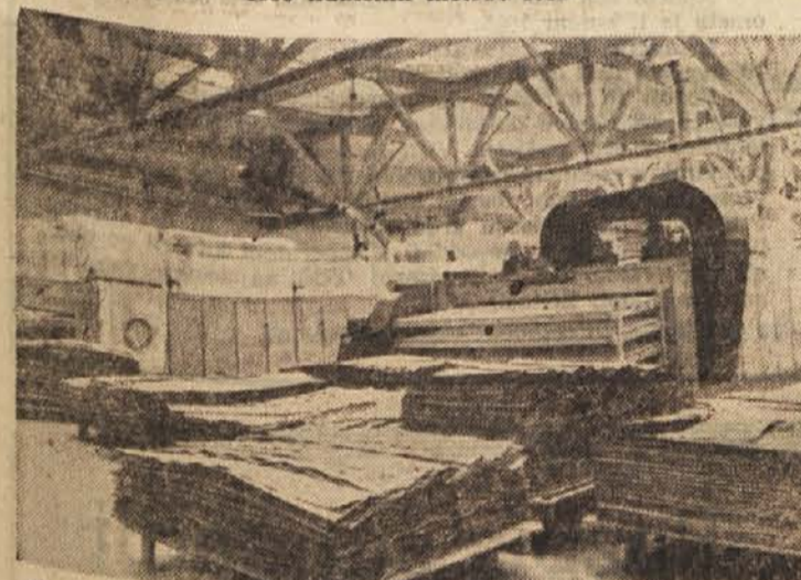
Slepi furnirji za vezane plošče gr edo iz luščilnega stroja v kanal-ske sušilnice, kjer se osuše
