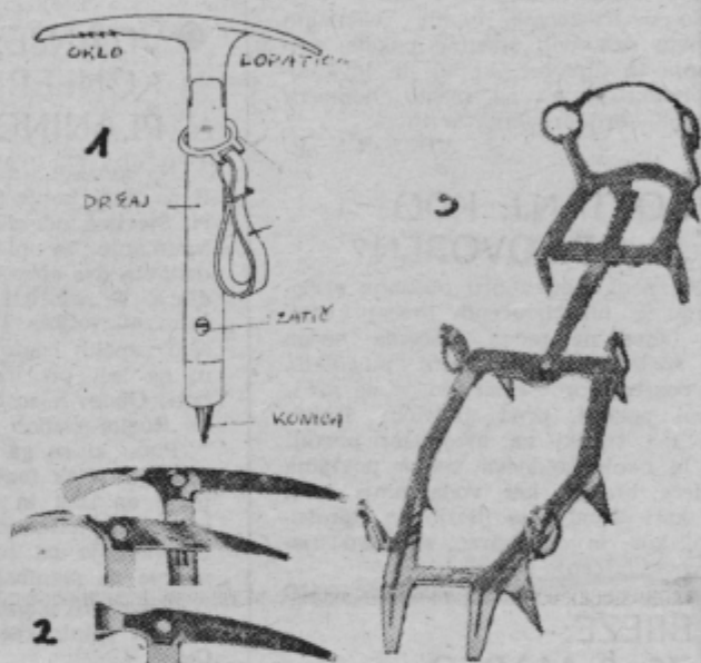
1 — cepin z obročkom, gajko in zatičem, 2 — dve obliki cepina in ledna bajla, 3 — dereze dvanajsterke s prestavljivo sredino — model Stubei
