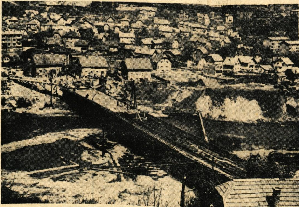
Most, ki bo povezoval Javornik z Blejsko Dobravo, že dobiva svojo podobo. Te dni so že začeli z betoniranjem cestišča. Potem bodo naredili še priključke ceste z obeh strani. Predvidoma bo most s priključki cest veljal 129 milijonov dinarjev
