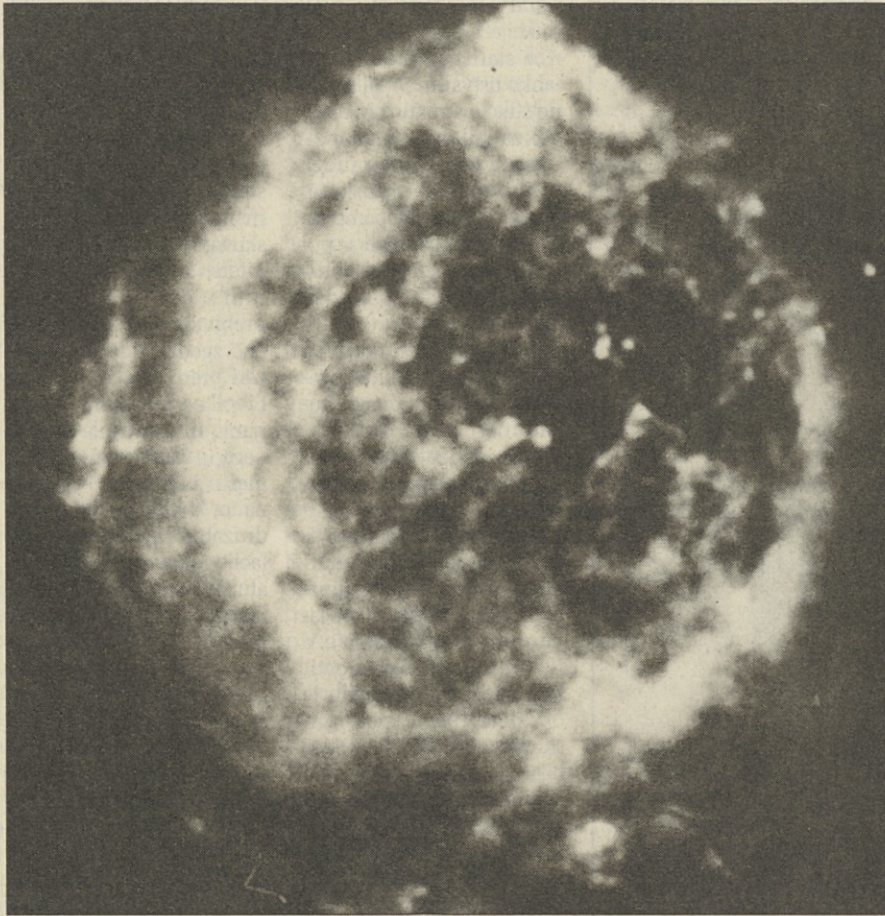
Ostanki eksplodirane zvezde; radijski vir Kasiopēja A (Foto: observatorij Mullard)
