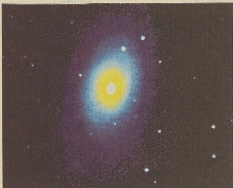
Supernova v galaksiji M81 - Obe sliki sta bili posneta z avtomatskim teleskopom na Astronomsko geofizikalnem observatoriju Golovec oddelka za fiziko FNT. Leva slika je bila posneta pred dvema letoma in na njej ni supernove. Desno nad jedrom galaksije sta dve svetli zvezdi in tretja sibejska. Ista trojica je vidna tudi na desni sliki, vendar je zelo blizu, levo od tretje zvezdice še svetlejša zvezda. Ta je supernova. Več o tem pojavu na str. 14.
