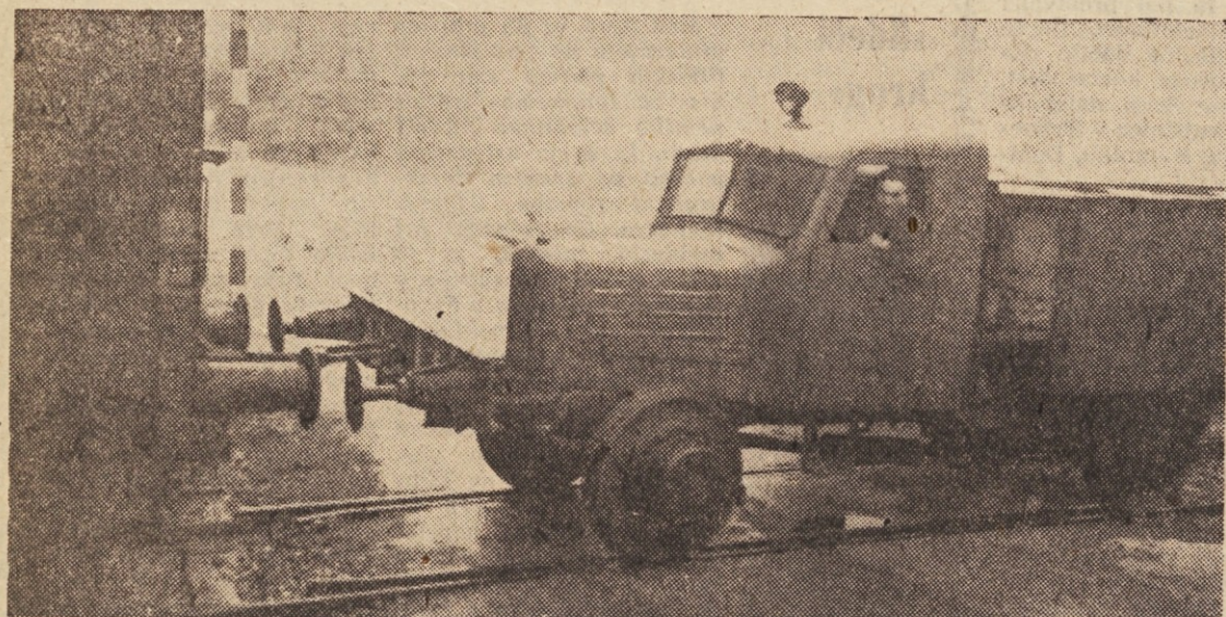
Utrudljivo in počasno premikanje na manipulacijskem tiru v kemični tovarni v Mostah je zamenjal sicer že odslužen kamion. Z domiselno rekonstrukcijo je tovarna usposobila star »MERCEDES« za vožnjo po železniškem tiru. S tem so dokaj pridobili na času, saj so premiki vagonov neprimerno hitrejši in tudi število ljudi, ki so bili zaposleni pri manipulaciji z vagoni, so s tem znatno zmanjšali.
