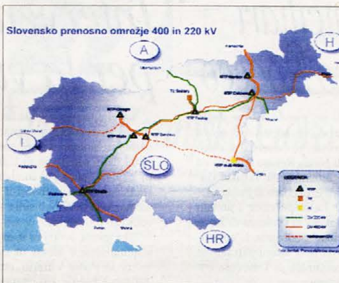
La rete di trasmissione elettrica della Eles con la previsione di tre nuovi elettrodotti, tra cui quello che unirà Okroglo a Udine
