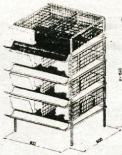
ETAŽNA KLETKA ZA PREPELICE
