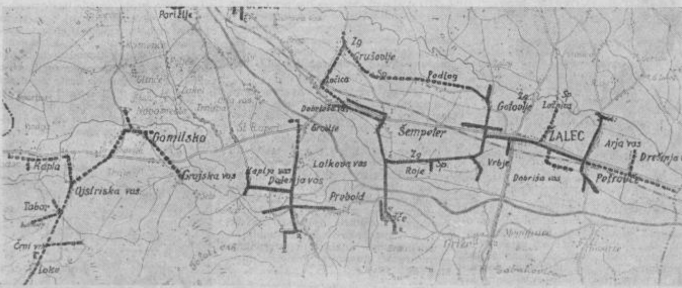
Tako bo speljan vodovod v žalski občini. Dela v prvi etapi so označena z debelo črto in bodo v glavnem zaključena že letos. Cez nekaj let ne bo več vasi v Savinjski dolini, ki ne bi imela vodovoda.
