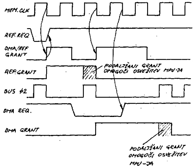
Slika 4. Časovni poteki pomembnejših signalov
