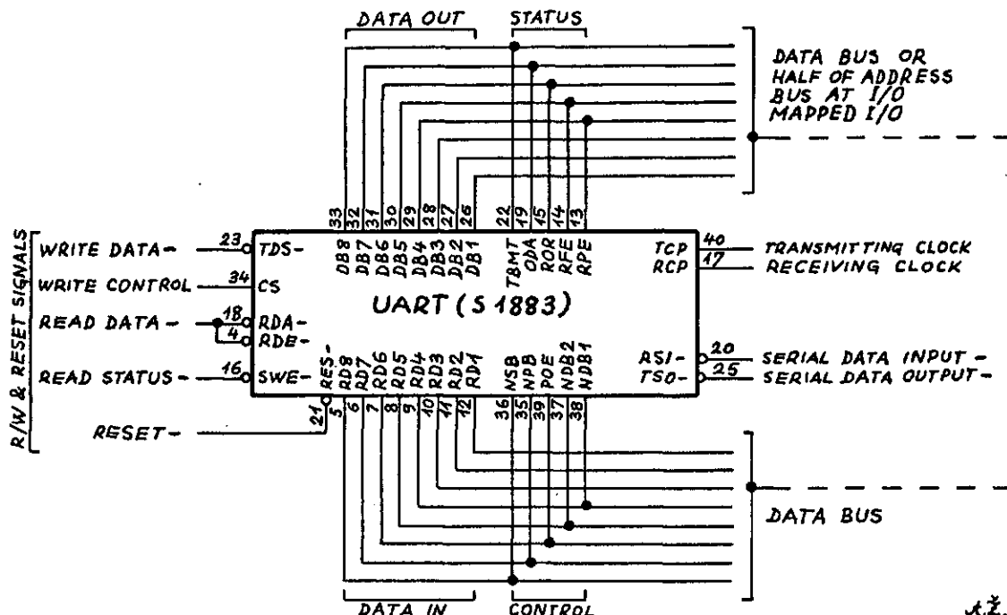
Slika 1. Integrirano vezje tipa UART (n. pr. S 1883), narisano v obliki (ustrezno povezano), ki je primerna za uporabo v mikro računalnikih (podatkovno, naslovno in krmilno vodilo).
