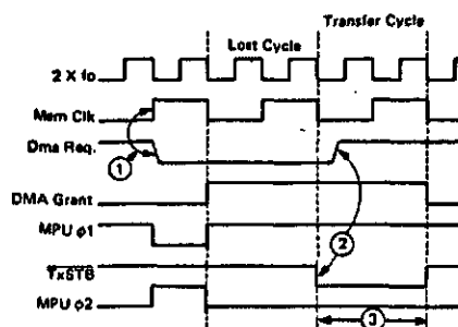
Časovni poteki signalov pri DMA prenosu. Dolžino DMA REQ. signala definira DMA kontroler (6844), kot funkcijo pomn. ure (1) in signala TxSTB (2), ki označuje, kdaj se je izvršil DMA prenos.
