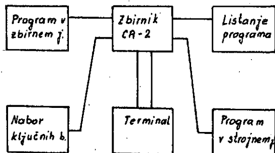
Sl. 2. Organizacija zbirnika CA-2 in potrebnih vhodnih ter izhodnih zapisov
