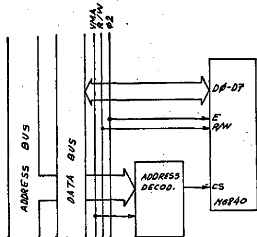
Slika 1. Uključivanje časovnika M6840 na sistemsko vodilo M6800.
