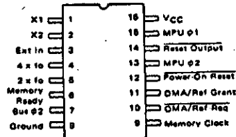
Slika 1. Razporeditev nožic za takti generator MC6875
