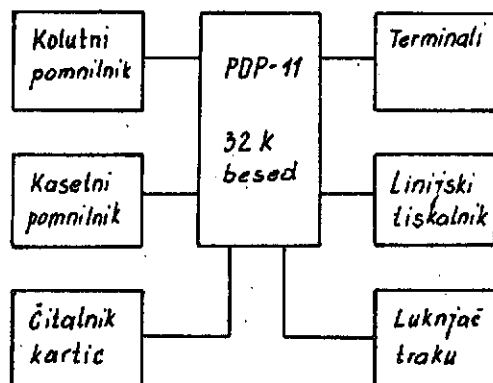
Sl. 1. Računalniški sistem za razvoj programske opreme
