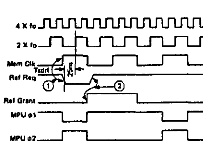
Časovni poteki signalov pri osveževanju dinamičnega pomnilnika.
