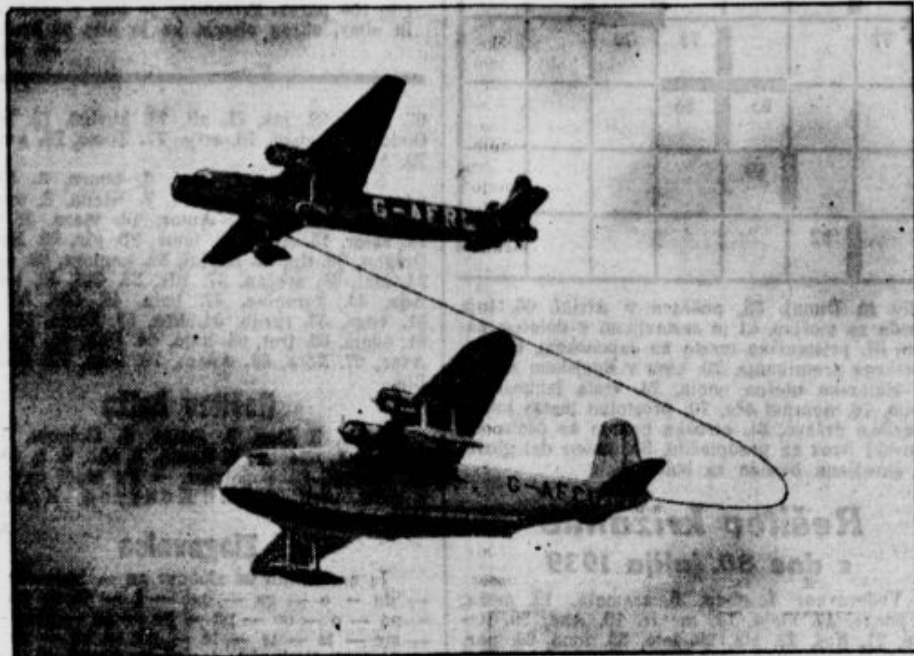
»Leteci tank« so preizkušali pri nekem čezoceanskem poletu nad Southamptonom. Angleski bombnik v zraku oddaja potniškemu letalu »Cabo« pogonski material. Obe letali sta v polni vožnji.
