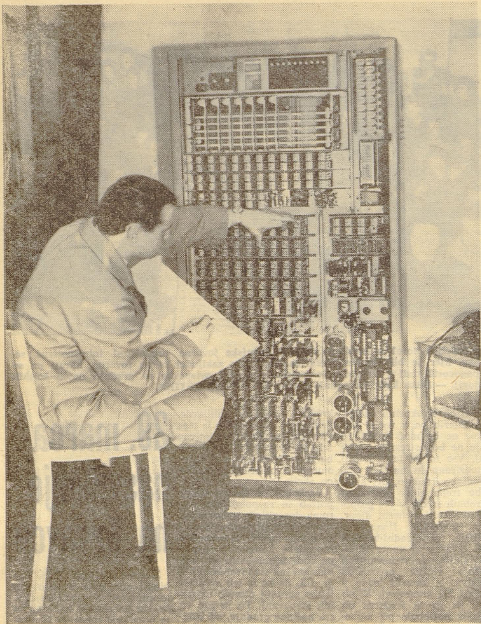
Takšna je naša nova ATC ISKRA 58 C 20, ki bo odigrala pomembno vlogo v telefonskem prometu na deželi
