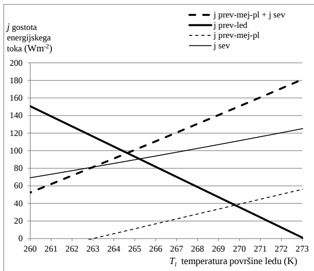
Slika 2. Prevajanje toplote skozi mejno plast in sevanje; presečišče debelejše neprekinjene krivulje (prevajanje skozi led) in debelejše črtkane krivulje (prevajanje skozi mejno plast in sevanje) je pri T_l = 264,5\text{ K} = -8,7\text{ °C} .
