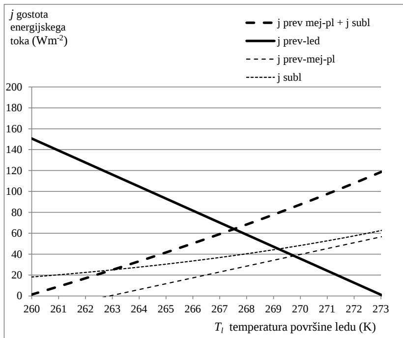
Slika 3. Če prevajanju skozi mejno plast dodamo gostoto toka sublimacijske toplote, je temperatura površine ledu (križišče debelejšše neprekinjene in debelejšše prekinjene črte) T_l = 267,5 \text{ K} = -5,7 \text{ }^\circ\text{C} – v primerjavi z zgolj prevajanjem skozi mejno plast za 2,3 \text{ }^\circ\text{C} nižja. Pri prejšnji grobi oceni o T_l = -5 \text{ }^\circ\text{C} torej nismo bili daleč od natančnejše določene vrednosti.
