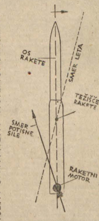
SL. 8. ZA STABILNOST RAKETE MED POLETOM SKRBI VRTLJIVO OBESENJE RAKETNEGA GONILA
