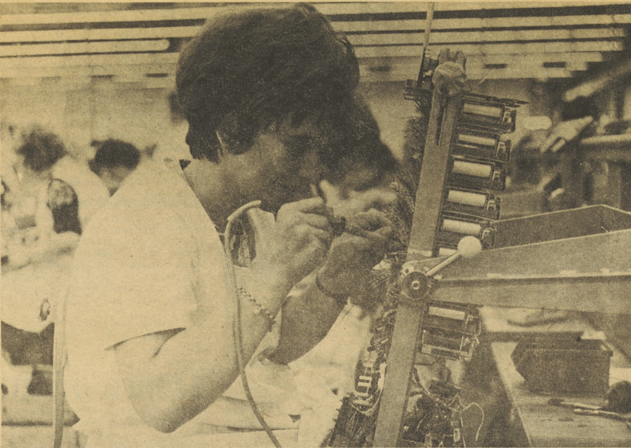
Nova linja telefonskih enot v tovarni telekomunikacij na Laborah — Kranj je že v teku. Slavnostna otvoritev tovarne bo 28. julija.
