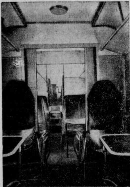
Pogled v notranjost letala »D 2500«: V dolgi kabini je za potnike 34 udobnih sedežev.
