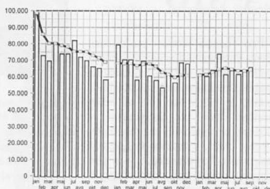
Pregled porabe pitne vode za leto 1997, 1998 in 1999
