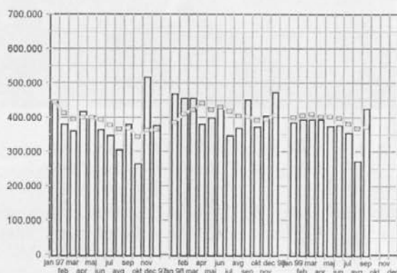
Pregled porabe hladilne vode za leto 1997, 1998 in 1999
