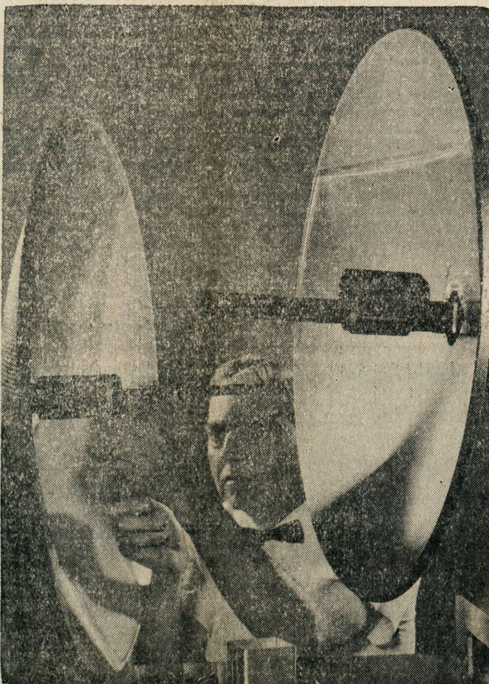
POGLED V DALJAVO — Slika kaže anteni radarja na jet letalih, ki je sposoben pogledati do 300 milj daleč in ugotoviti nevarne spremembe vremena. Elektronski inženir na mešča anteni. Te vrste radarja bodo nujne za nadzvočna potniška letala bodočnosti.
