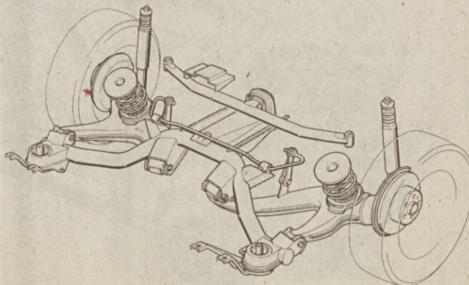
...zadnja prema - trikotna prečna vodila
