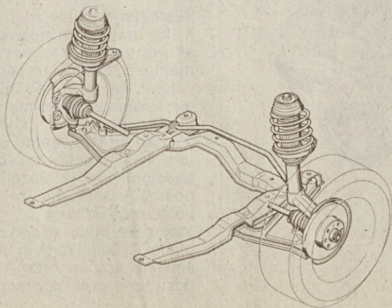
Prednja prema - posamične obese in nihajoča vodila...
