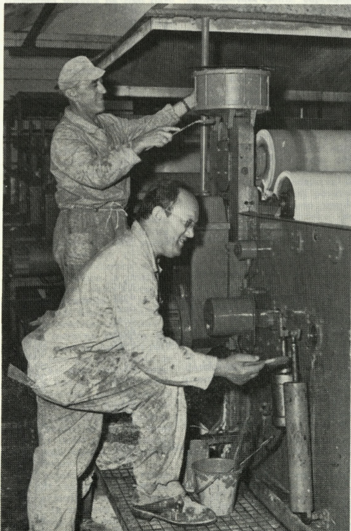
Pleskarja Franc Trilar in Peter Sušnik pri pleskanju ohišja mercerizirnega stroja
