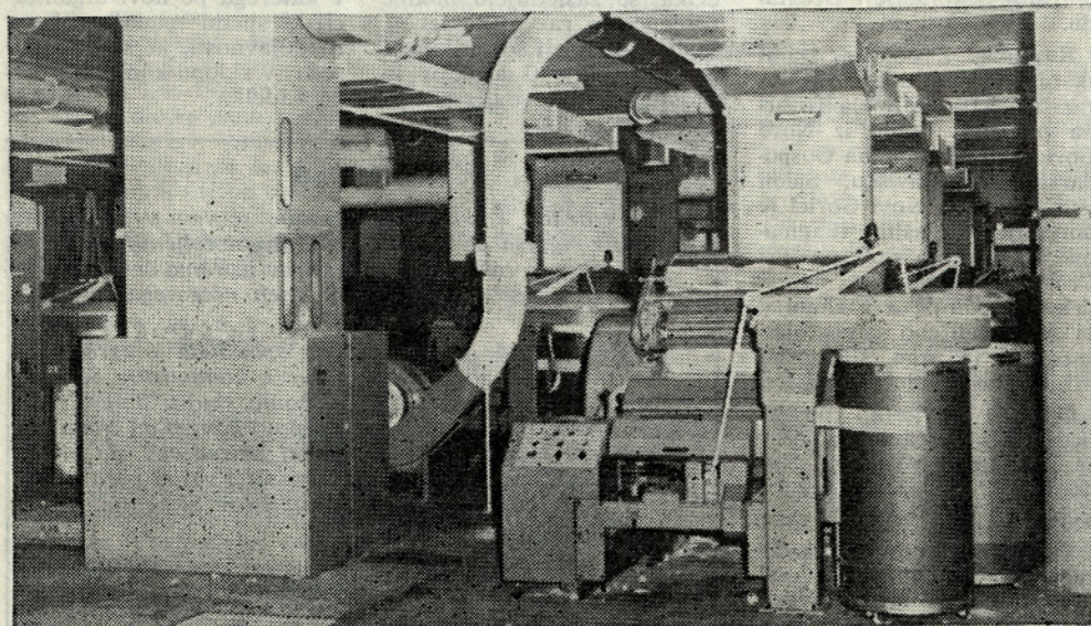
Novi mikalniki v predilnici
