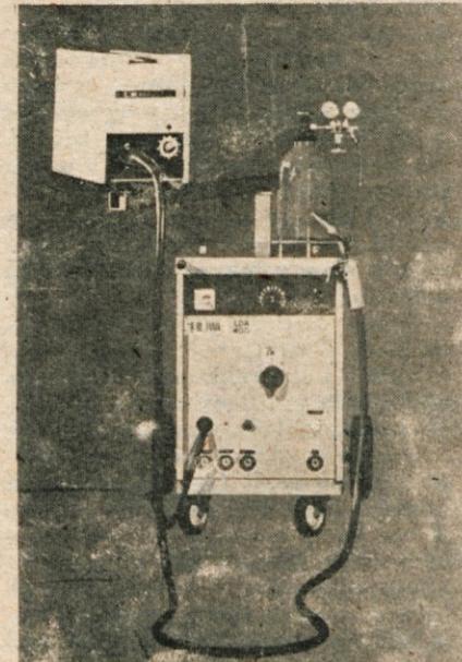
A 10-275 naprava za polavtomatsko varjenje A 10-275 in A 10-400
