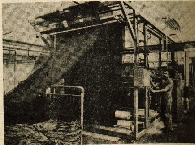
Kranj — Že nekaj časa poskusno obratuje novi plastificirni stroj, s katerim bo Zvezda popestrila svojo ponudbo medvlog. — Foto: F. Perdan
