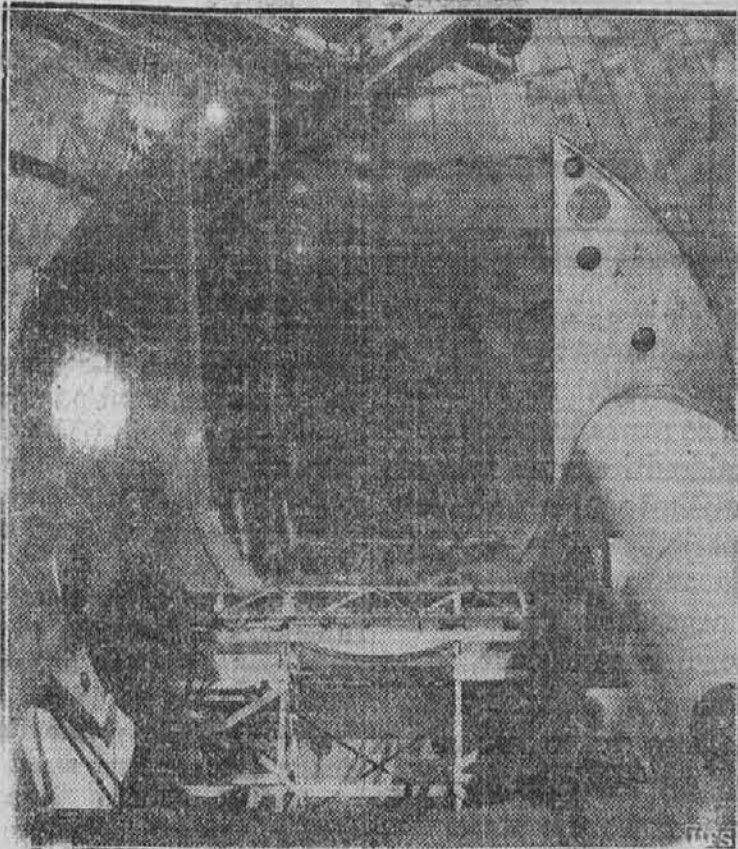
V Palomer Mountain zvezdarni v Kaliforniji je novi daljnogled popolnoma dogotovljen in zdaj čakajo le še, da bo končano delo z brušenjem ogromnega zrcala, ki meri 200 inčev. Ta daljnogled bo odkril zvezdoslovem nova čudesa vesolja.
