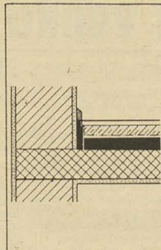
TOPLOTNA IN AKUSTIČNA IZOLACIJA PODOV
