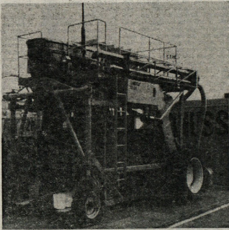
Sistem vertikalnega stresanja. Na sliki so dobro vidne cevi za odvajanje drozge v posebne tanke
